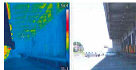
同日同時 塗装済み 笠間DC(茨城県)サーモグラフィー画像
